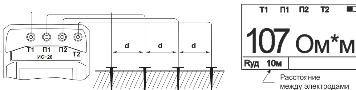
Рисунок 2.3.8 - Схема подключения и вид индикатора при измерении удельного сопротивления грунта
